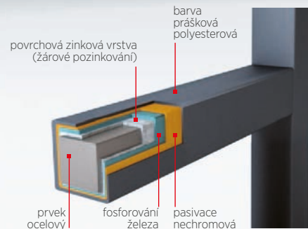
Průřez prvkem zabezpečený v systému DUPLEX
